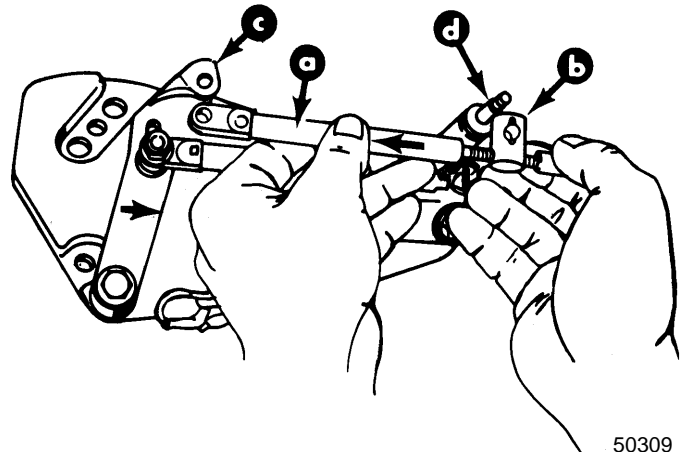
a - End Guide b - Brass Barrel c - Shift Lever Clevis Pin Hole d - Stud
